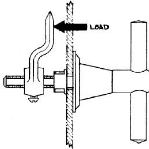
Nº 68 FASTENER - 100 SERIES
